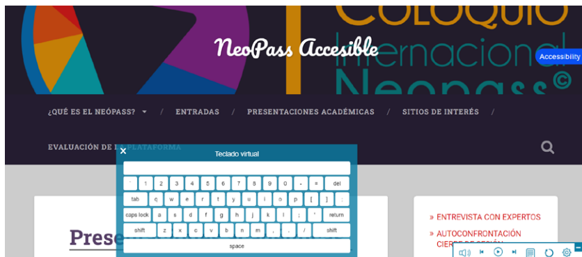
Figura 5. Teclado virtual
