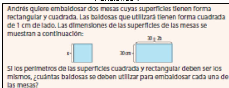
Figura 4 – Problema propuesto en la sección “Aplico mis aprendizajes” de la Unidad 2 “Álgebra y Funciones”.
