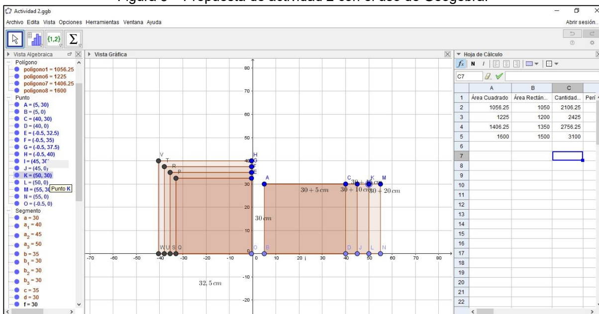
Figura 5 – Propuesta de actividad 2 con el uso de Geogebra.
